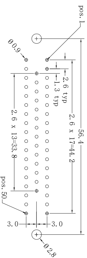
P.C.B Layout
